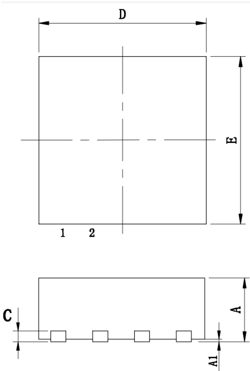
封装图 (DFN2X2_8L)
